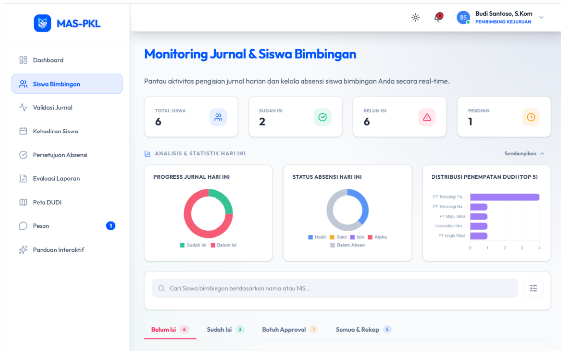
Gambar 7.2: Daftar Siswa Binaan Guru Pembimbing dengan Fitur Push Pengingat Jurnal & Reset Sandi
