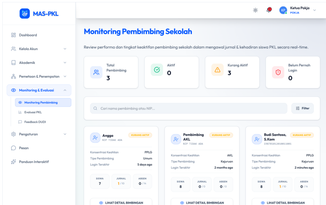
Gambar 6.7: Antarmuka Monitoring Aktivitas Guru Pembimbing dan Formulir Catatan Evaluasi Pokja
